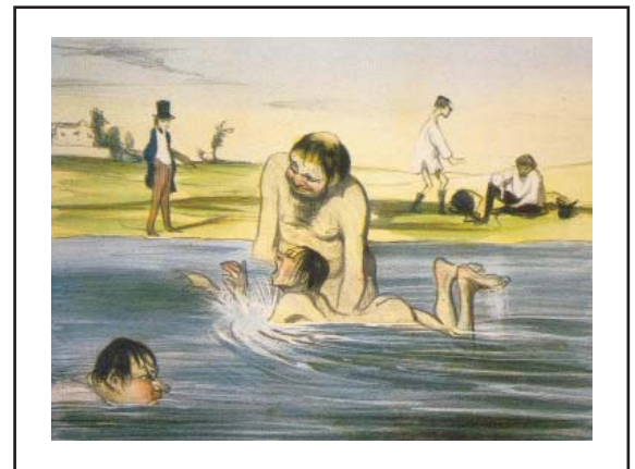
FIGURA 3. ¡Aquí tenéis un pequeño diablillo delfín! Siempre estaría en el agua si no lo sacáramos
