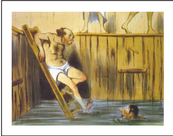
FIGURA 5. Venga abuelo, venga con nosotros al "caldo"
