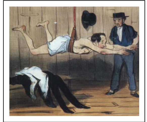
FIGURA 2. Ejercicio en seco. Si ha realizado este ejercicio durante tres meses de forma ininterrumpida y es trasladado sin miramientos a la "categoría de pez"... entonces incluso el más tímido puede demostrar su arte natatorio sin ningún temor
