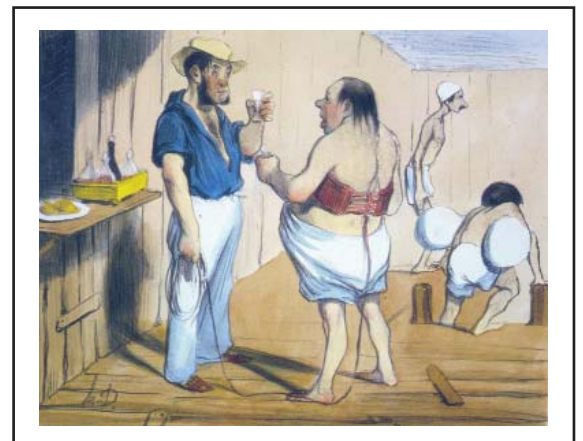
FIGURA 4. Escúcheme, usted esta en la mejor edad. ¡Cuando un hombre es tan elegante y se mantiene perfectamente sobre el agua, su monitor se alegrará! Tómese seriamente mis clases, beba de cuando en cuando un par de vasitos y podrá competir con todos!
